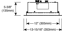
300-HWILF/D4
